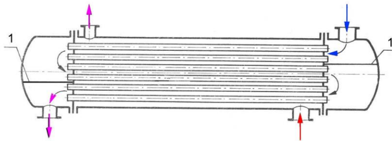
Rys. 1-2. Wymiennik płaszczowo-rurowy, równoległy prądowy, trójdrogowy, przepływ mieszany. 1 – przegroda.
