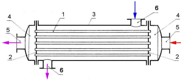
Rys. 1-1. Wymiennik płaszczowo-rurowy, równoległy prądowy, jednodrogowy, współprądowy. 1 – rurka, 2 – dno sitowe, 3 – płaszcz, 4 – pokrywa, 5 – króciec, 6 – króciec.
