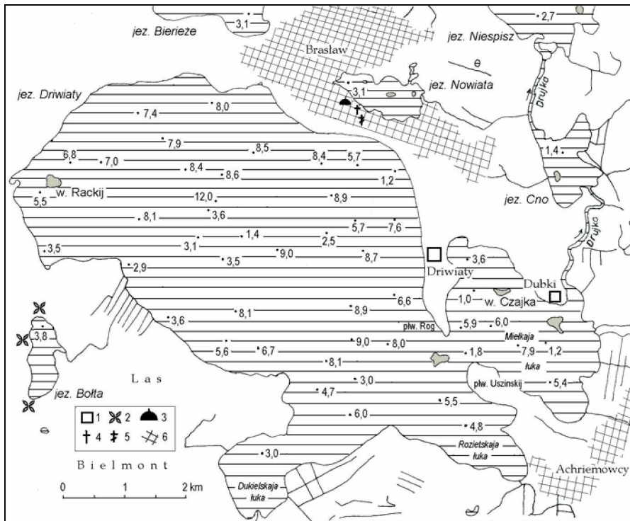
Rys. 10. Jez. Driwiaty i tereny bezpośrednio do niego przyległe (wg: Nacionalnyj park „Braślowskije oziara”... , 2007 – uzupełniony):
