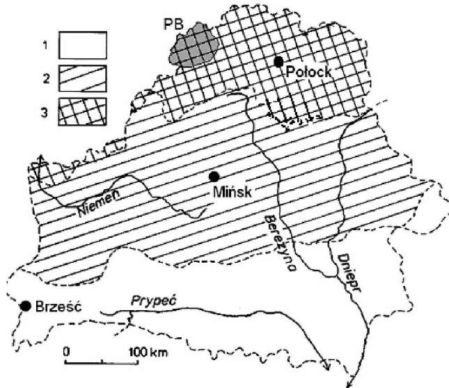
Rys. 1. Lokalizacja Pojezierza Brasławskiego (PB) na tle zasięgów zlodowaceń wg Atlas Respubliki... , 1998:
