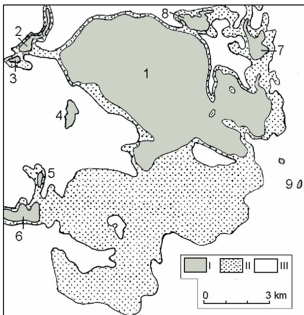
Rys. 15. Zanikanie jezior brasławskich (fragment rysunku wg J. KONDRACKIEGO, 1938):
