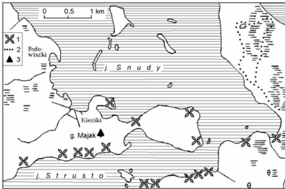
Rys. 20. Punkt widokowy góra Majak na półwyspie między jeziorami Strusto i Snudy (wg: Nacjonalnyj park... , 2007): 1 - pola namiotowe, 2 - ścieżka ekologiczna „Mieź-oziornyj” (Mieź-jeziorna), 3 - punkt widokowy
