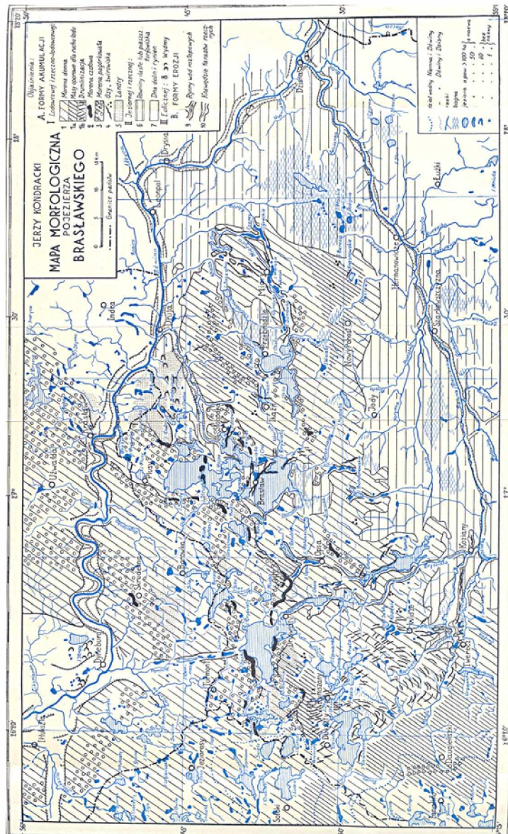
Rys. 7. Szkic geomorfologiczny Pojezierza Braślawnskiego wykonany przez J. KONDRACKIEGO (1938)
