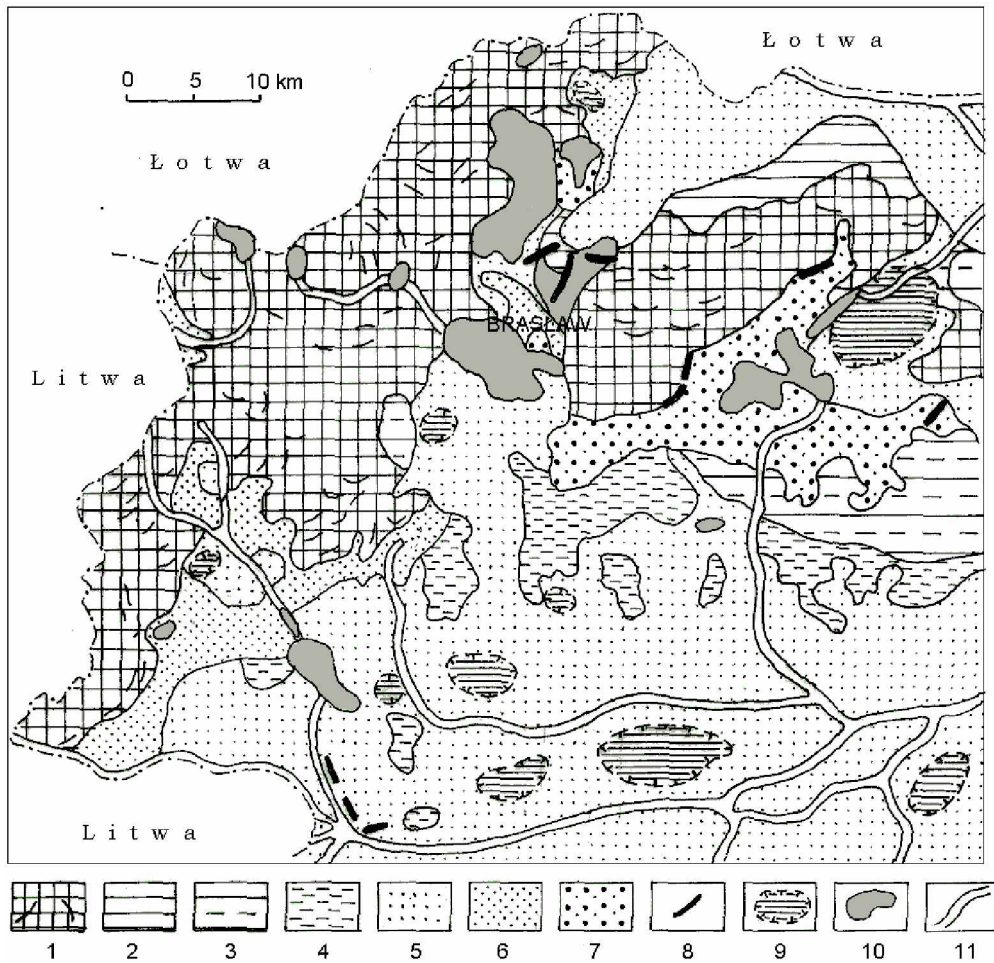
Rys. 6. Główne formy rzeźby analizowanej części Pojezierza Braślawskiego (wg Geomorfologicznej karta... , 1990 - uproszczony):
