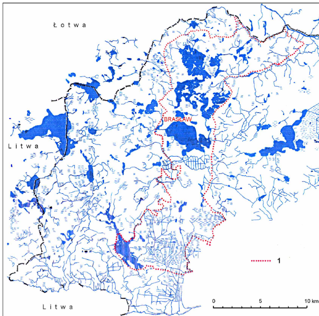
Rys. 8. Sieć hydrograficzna (bez nazw własnych obiektów) Pojezierza Brasławskiego (zestawiono na podstawie: KONDRAČKA, 1938; Nacjonalnyj park „Brasławskije ożiora” , 2007, 2009): 1 – granice Parku Narodowego (Jeziora Brasławskie)
