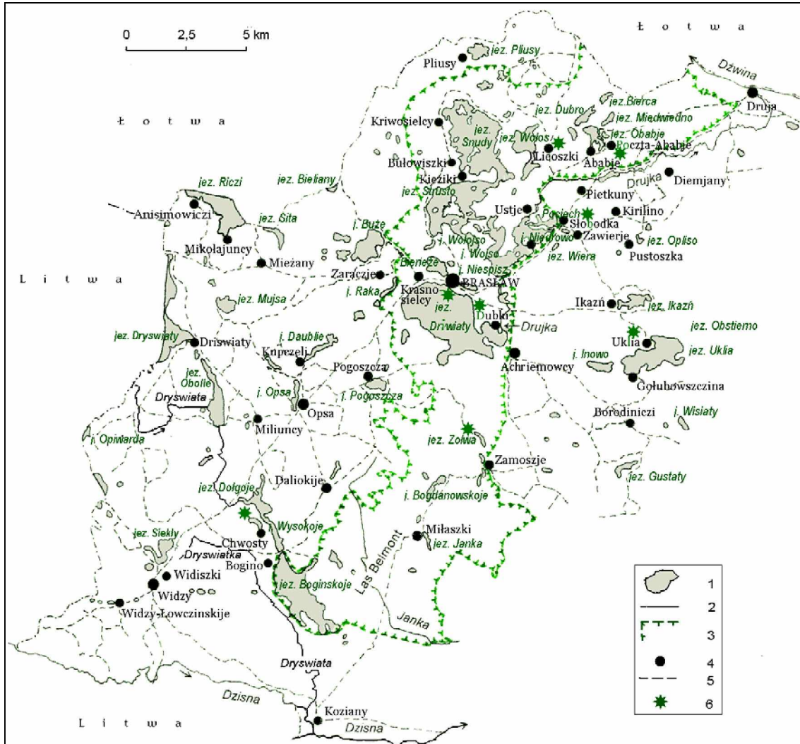
Rys. 9. Wybrane obiekty turystyczne na Pojezierzu Braślawskim (wg: Nacjonalnyj park „Braślawskie jeziora”... , 2007; nazwy własne obiektów – wg tego samego źródła, z wyjątkiem nazw rzek Dźwina i Dyzna oraz nazw państw):
